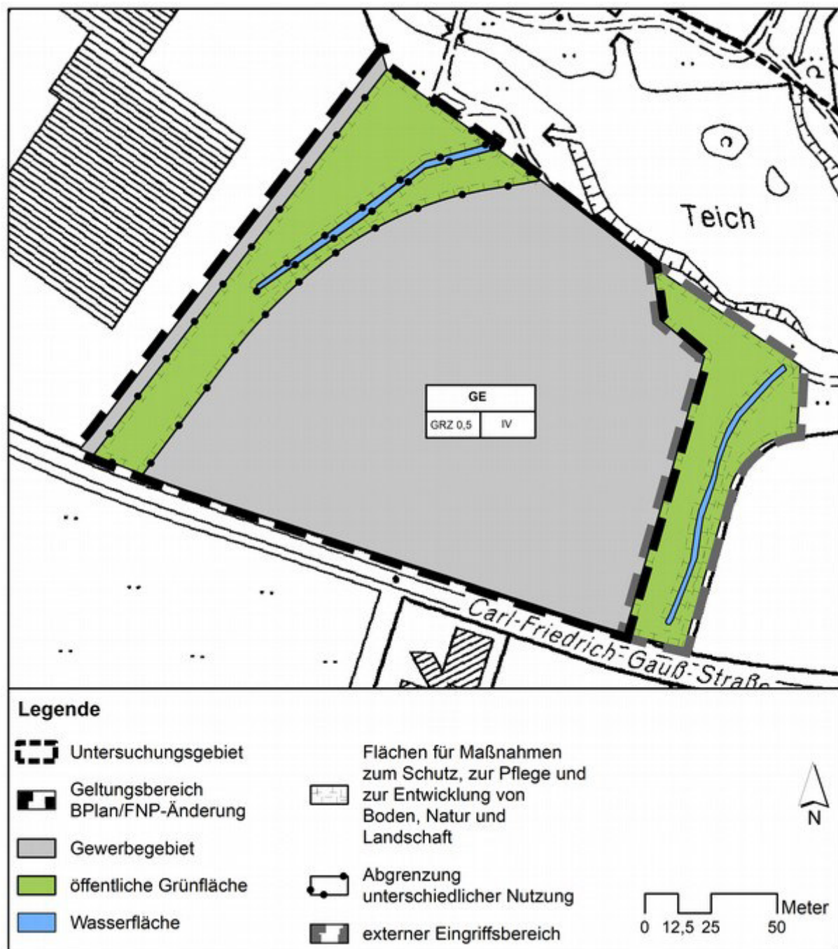
Abbildung 6: Bebauungsplan GES 118
